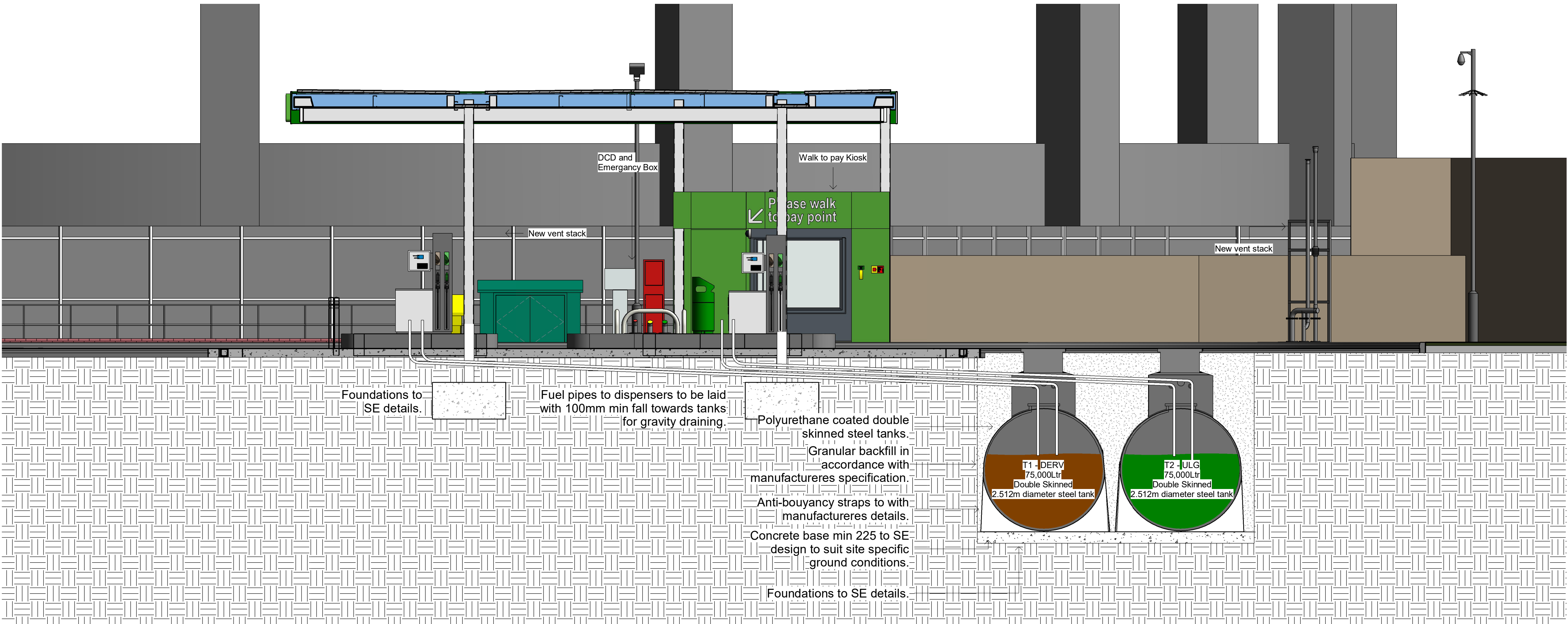
Long site section 1 : 50
