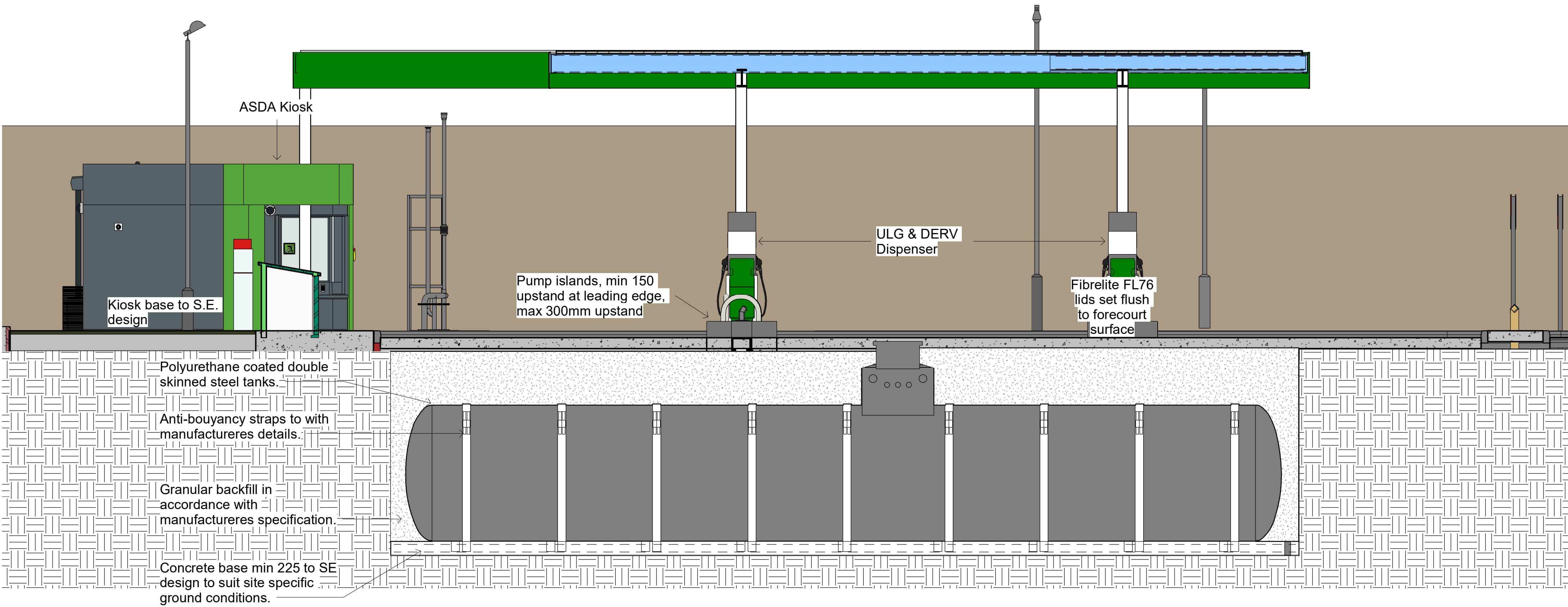
Site cross section 1 : 50
